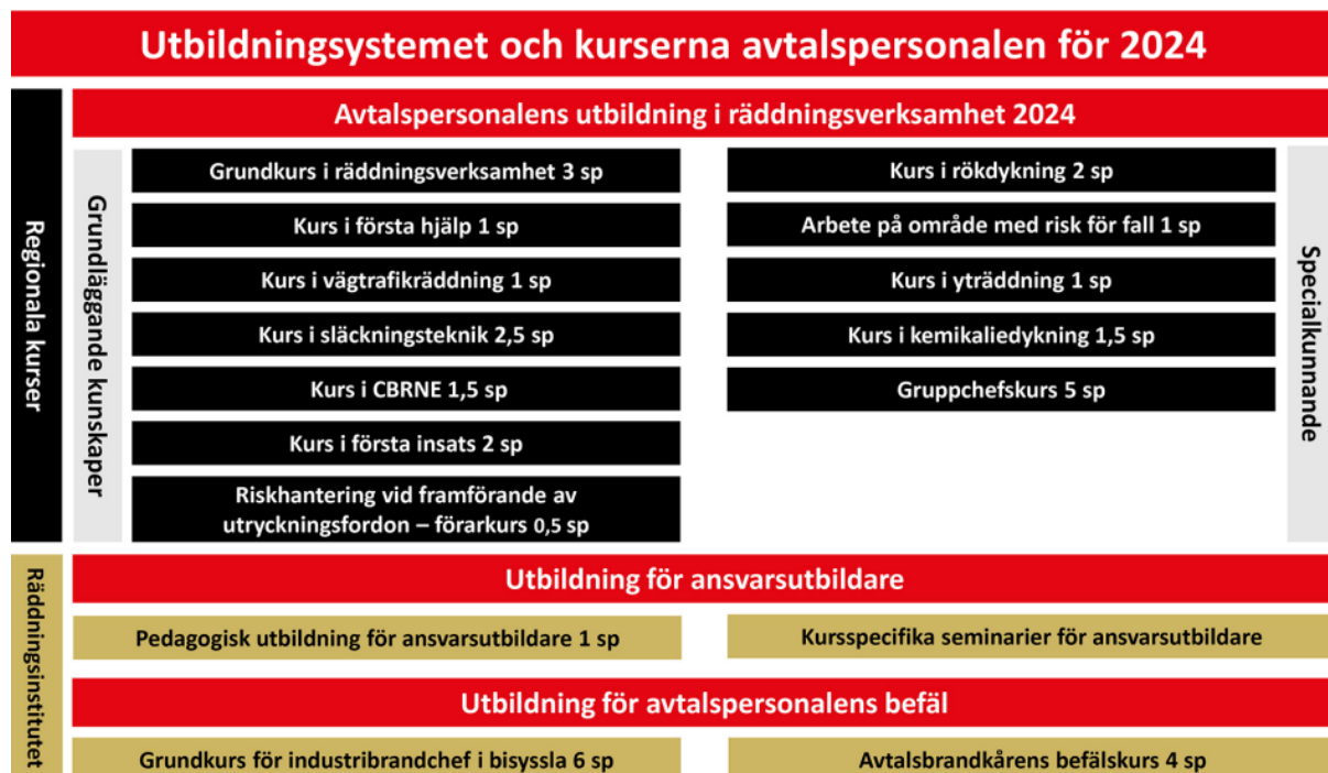
Bild 2 Utbildningssystemets kursschema
